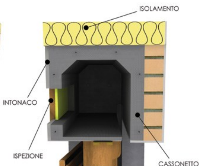
PARTICOLARE CASSONETTO
